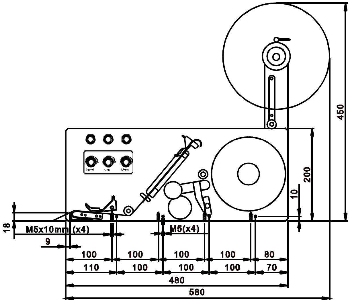
FIGURA 2 (vista laterale)
