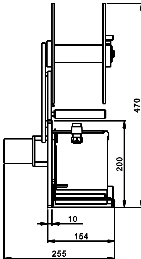
FIGURA 3 (vista frontale)
