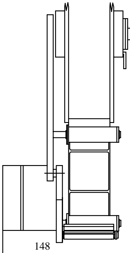
FIGURA 3 (vista frontale)
