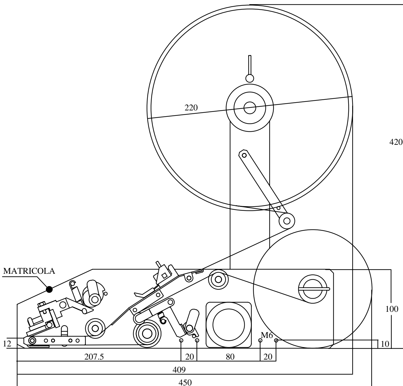
FIGURA 2 (vista laterale)
