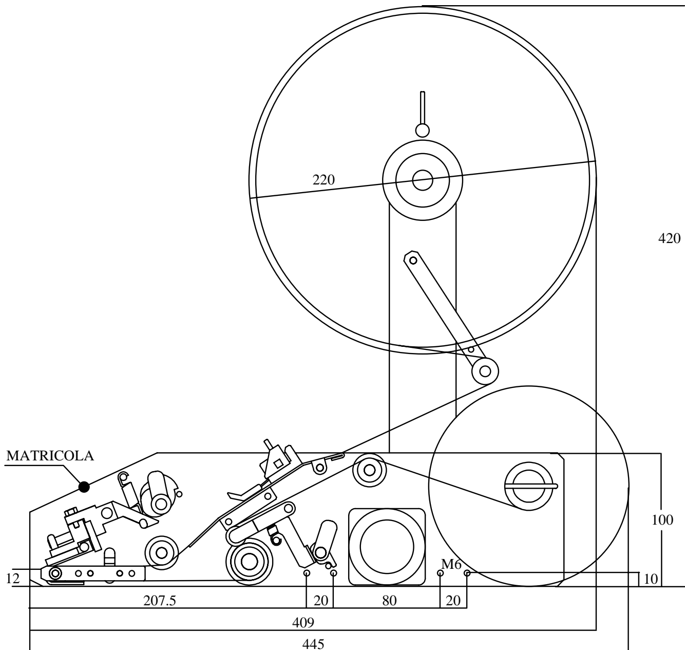
FIGURA 2 (vista laterale)
