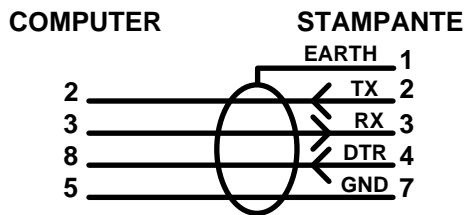
CONNETTORE COMPUTER A 9 PIN
